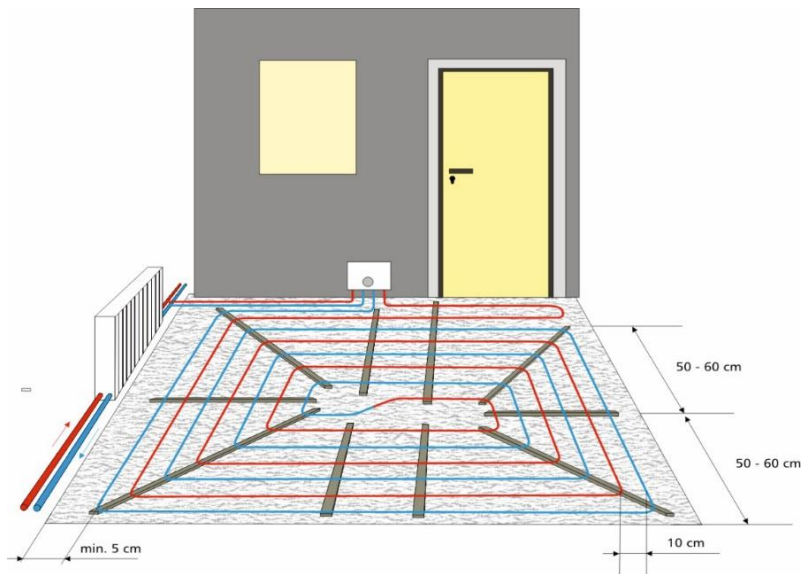
FLEXIRO Dünnbett Fußbodenheizung, Verlegeform: spiralförmig
