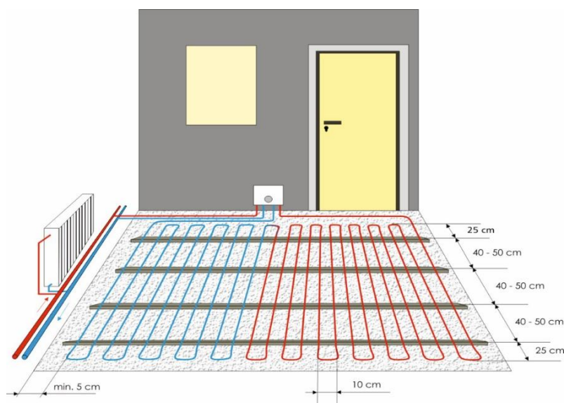
FLEXIRO Dünnbett Fußbodenheizung, Verlegeform: mäanderförmig
