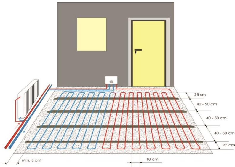
FLEXIRO Dünnbett Fußbodenheizung, Verlegeform: mäanderförmig
