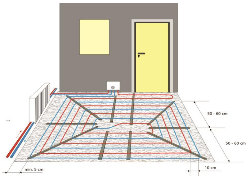
FLEXIRO Dünnbett Fußbodenheizung, Verlegeform: spiralförmig
